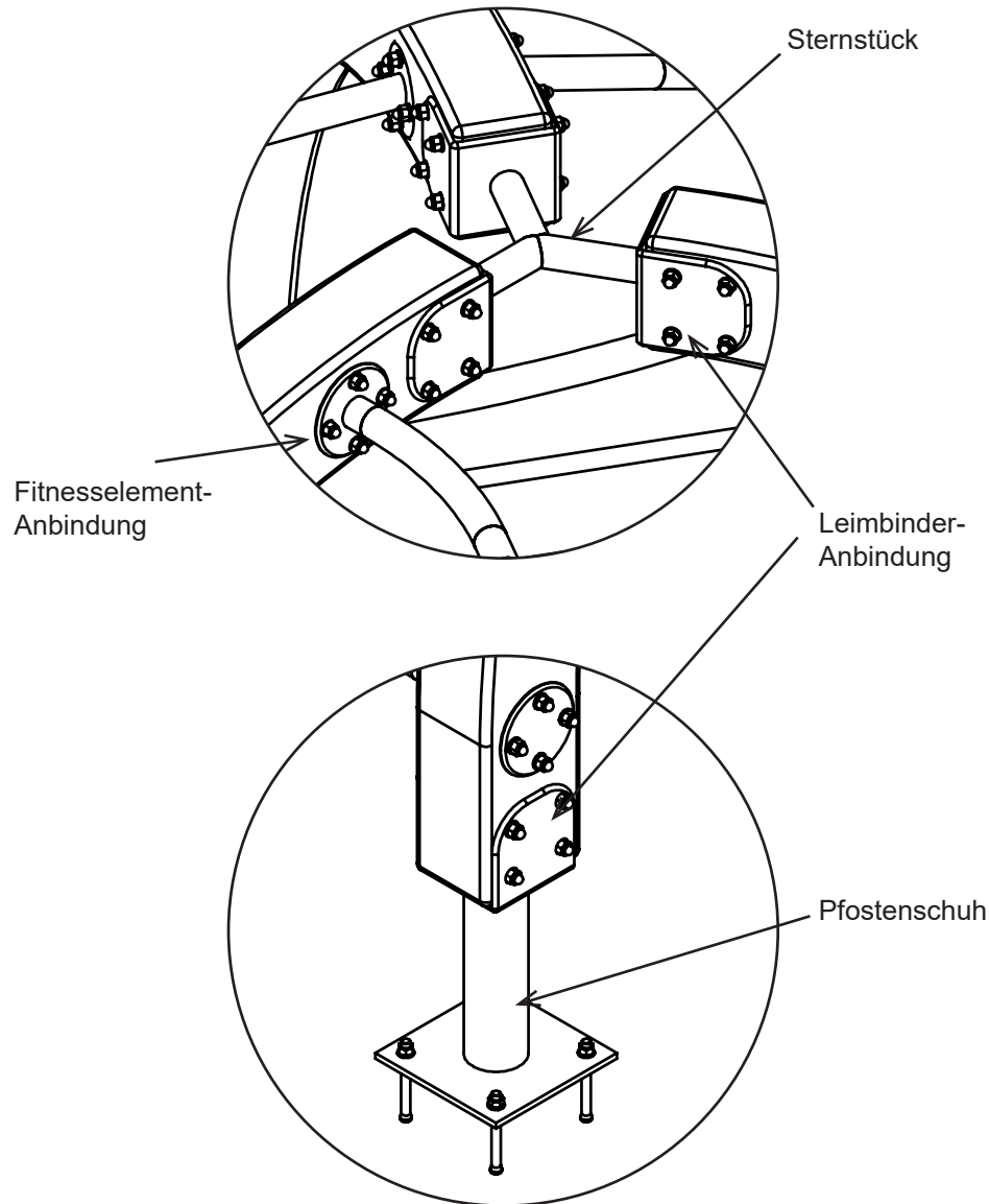
Skizze 3: Anbau Einzelemente
